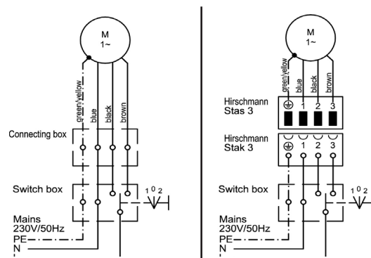
Fig. 4 Circuit diagram VariEco S-K mit 230 V / 50 Hz
