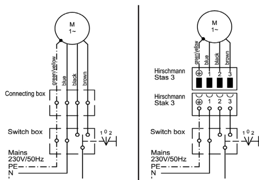
Fig. 4 Schema elettrico di VariEco S-K con 230 V / 50 Hz
